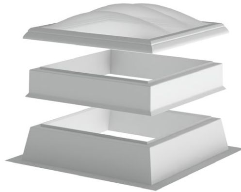
Abb. 2 – Lichtkuppel F100 W mit GFK Aufstockelement
